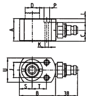
CLF50-10 - CLF450-15
