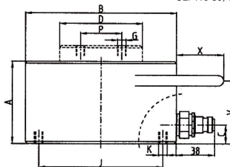
CLF450-40 - CLF2000-16
