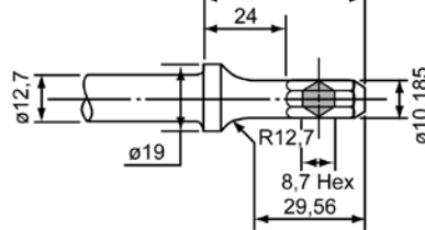
Sechskantschaft
