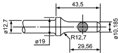
Rundschaft
