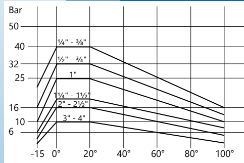
Druck- und Temperaturdiagramm
