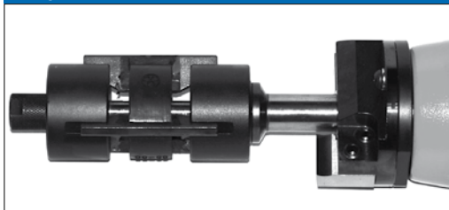
Spannfutter mit Schneidmesser (Bit)
